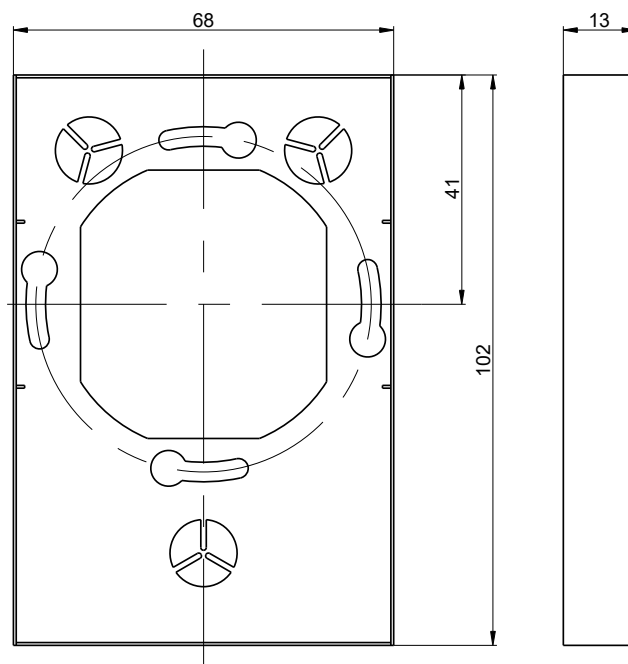
Montageplatte
