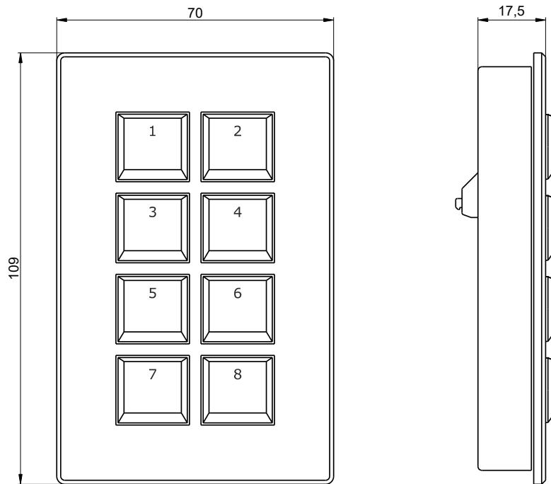
Montageplatte
